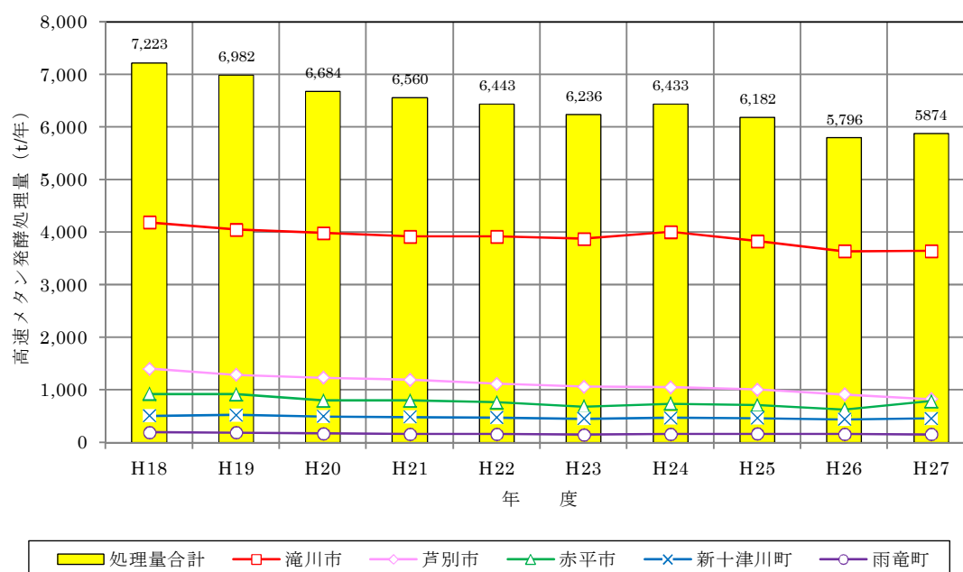
図 2.1.4 高速メタン発酵の自治体別処理量の実績推移
