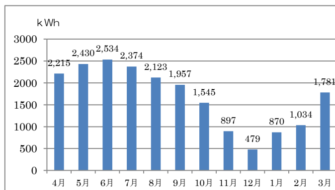
図 6 滝川高校における太陽光発電実績
