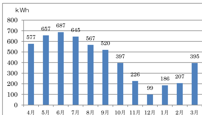
図 7 札幌地方検察庁滝川支部における太陽光発電実績
